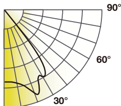
SPFTR6-LEL9035-KDIM010-UNV-WD-ADR6CC
