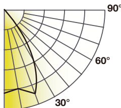
SPFTR6-LES9730-KDIM010-UNV-MD-ADR6CC
