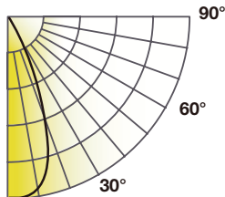
SPFTR6-LEL9035-KDIM010-UNV-NR-ADR6CC
