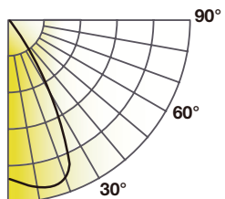
SPFTR6-LEL9035-KDIM010-UNV-MD-ADR6CC
